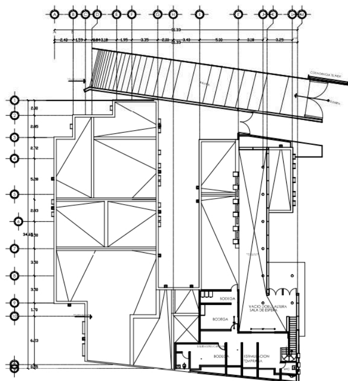
PLANTA ALTA
