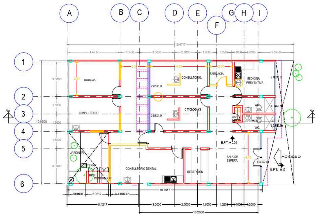
PLANO ARQUITECTONICO
