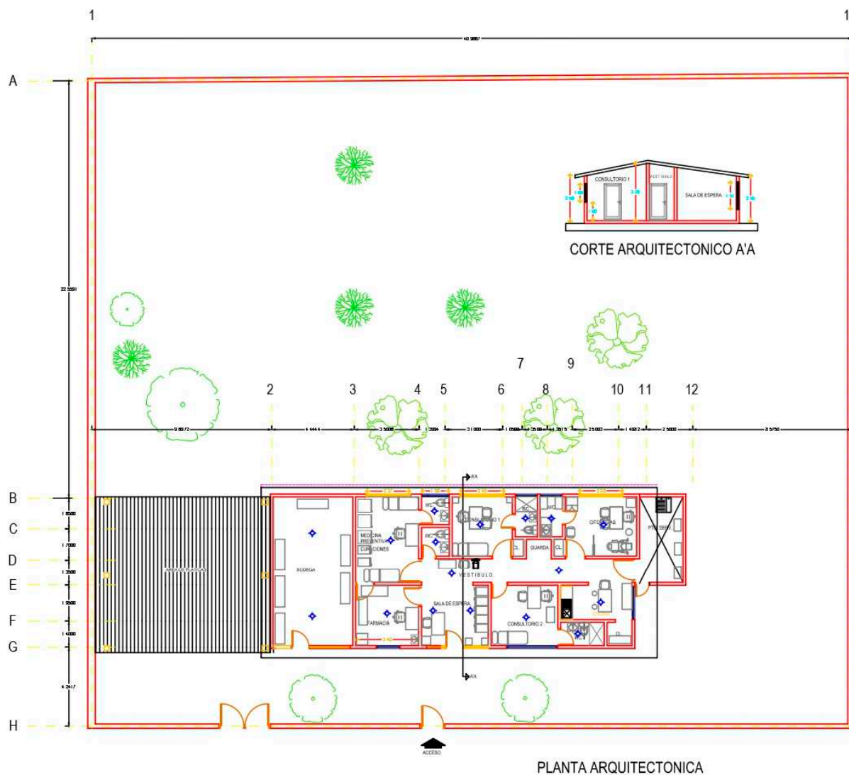
PLANTA ARQUITECTONICA
